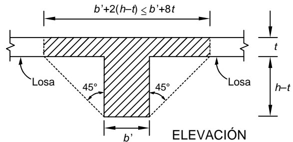
Figura 2.3 Ejemplos del tramo de losa que debe considerarse en el cálculo de A_{cp} y p_{cp}
